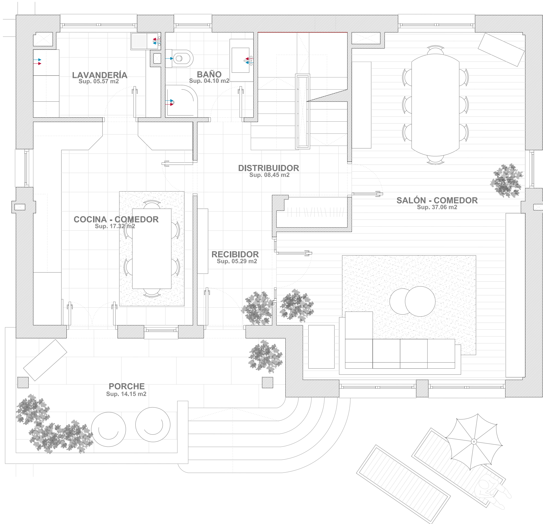
PLANTA PRIMERA
