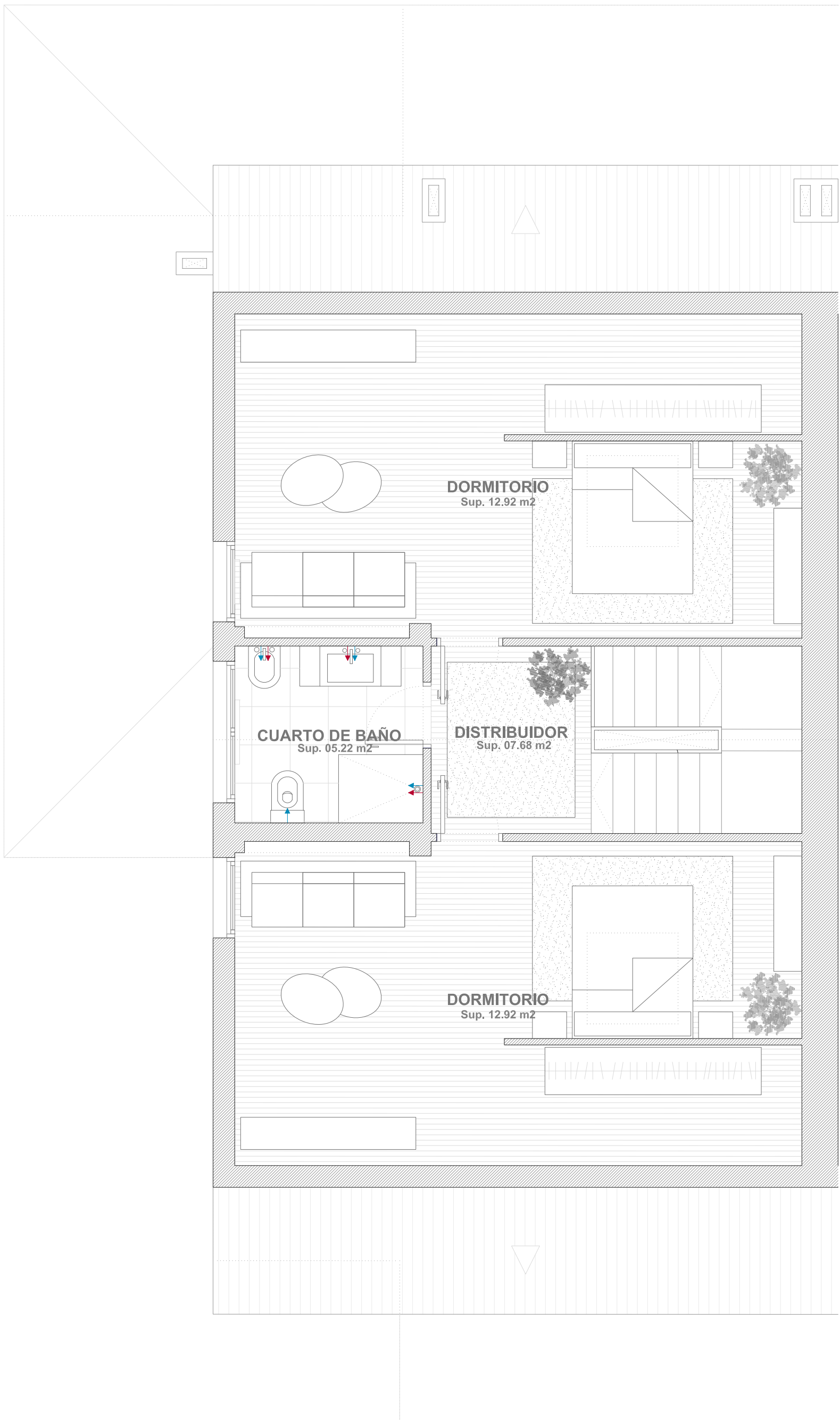
PLANTA ALTA
