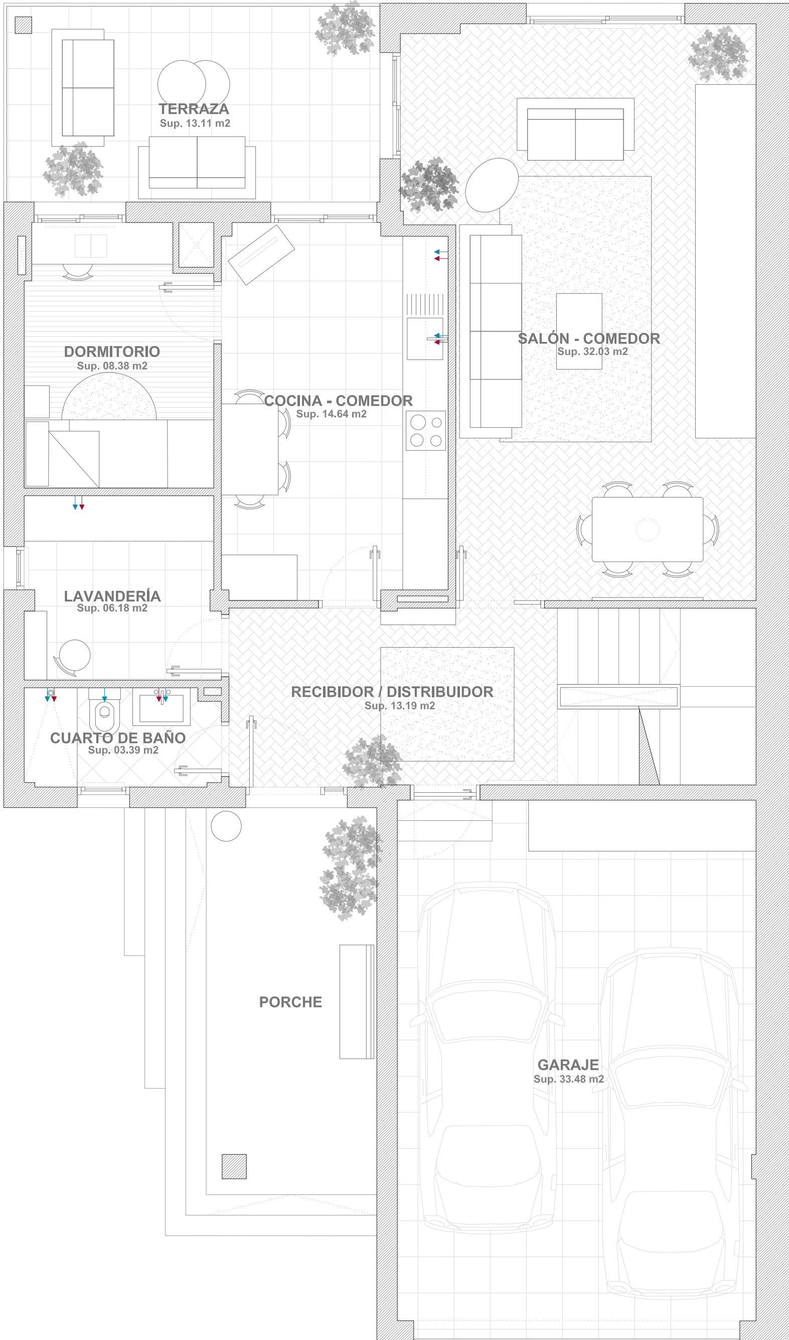
PLANTA BAJA
