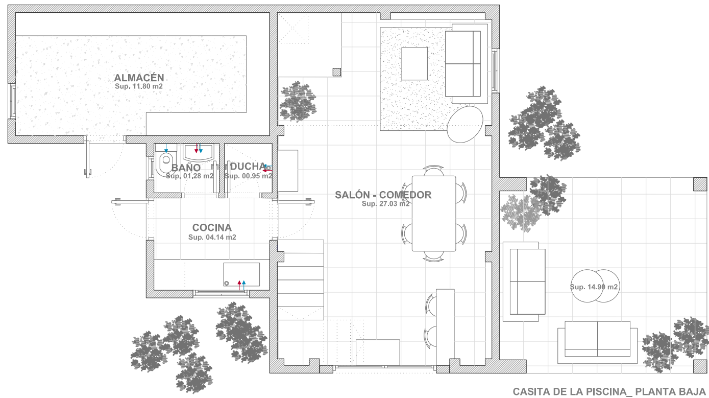
CASITA DE LA PISCINA_ PLANTA BAJA
