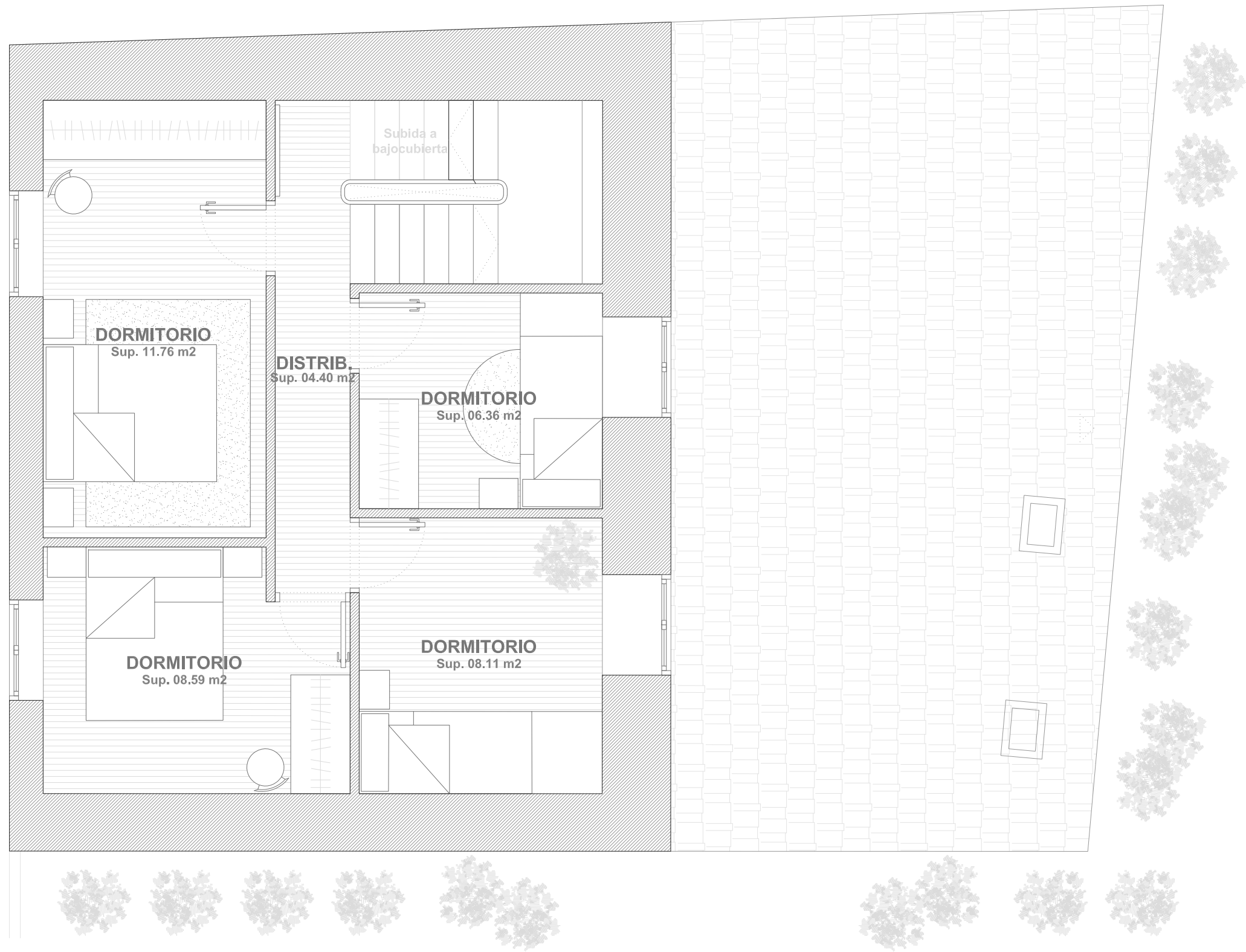
VIVIENDA PRINCIPAL_ PLANTA ALTA
