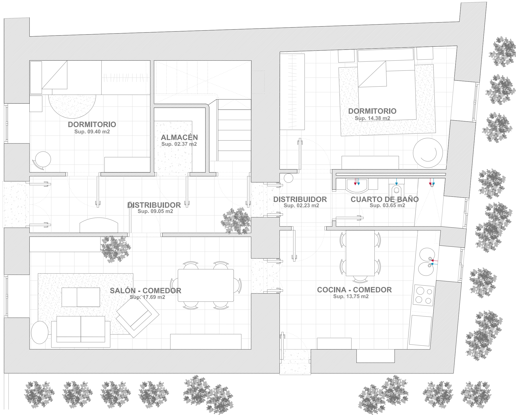
VIVIENDA PRINCIPAL_ PLANTA BAJA
