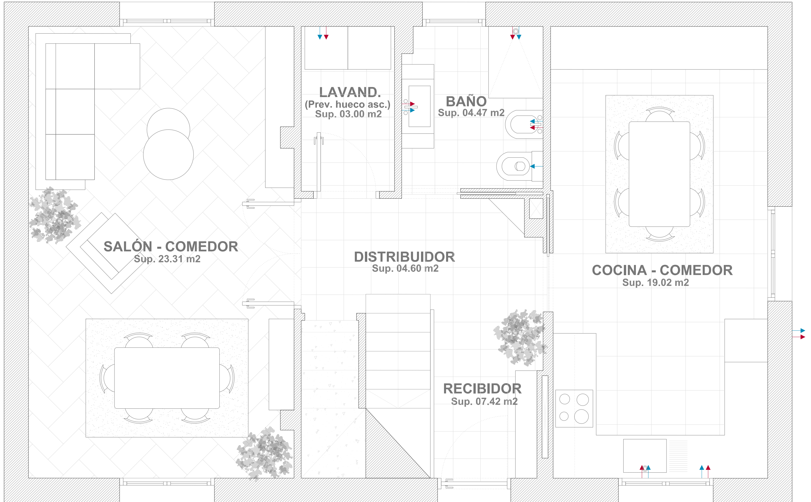
PLANTA BAJA
