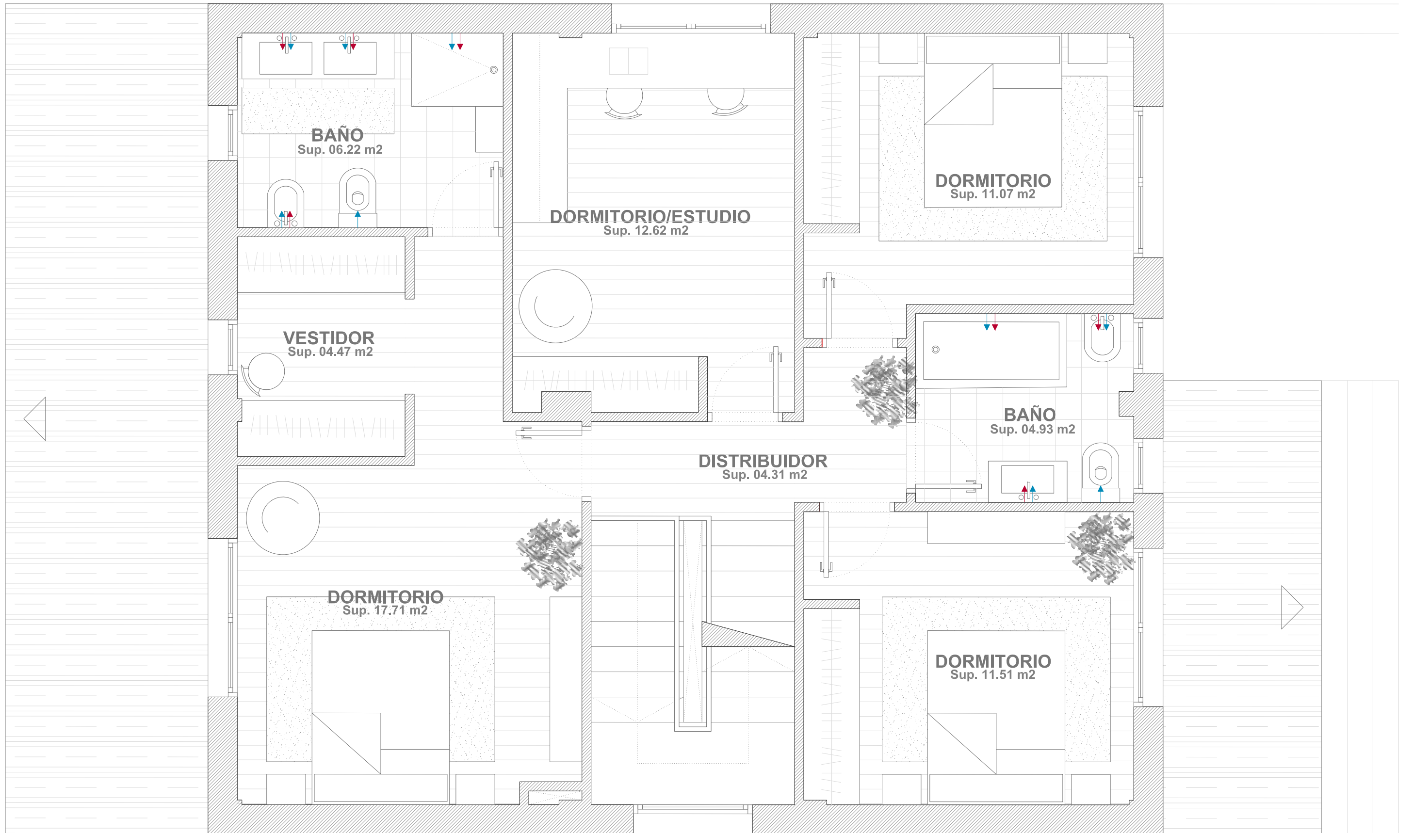
PLANTA ALTA
