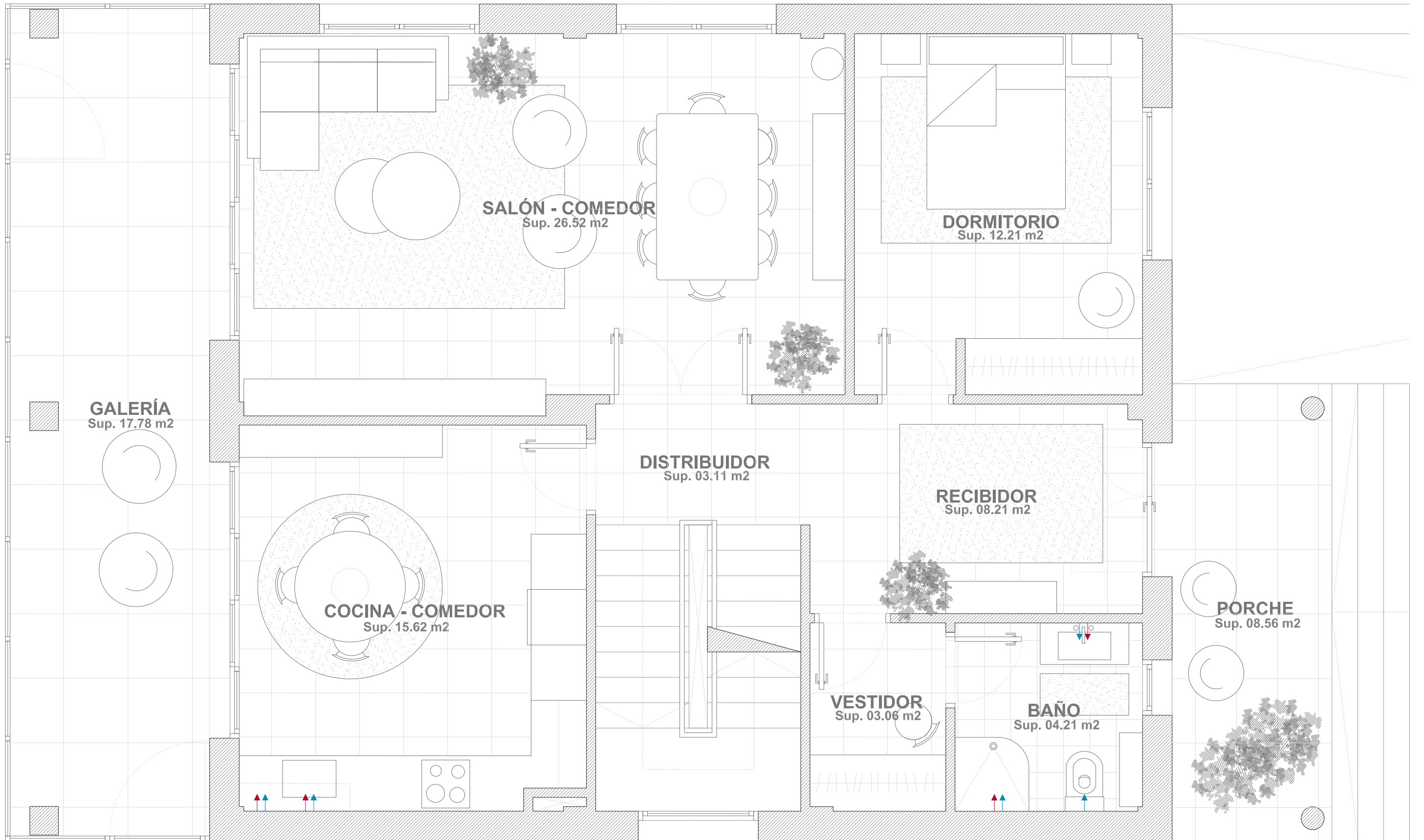
PLANTA BAJA
