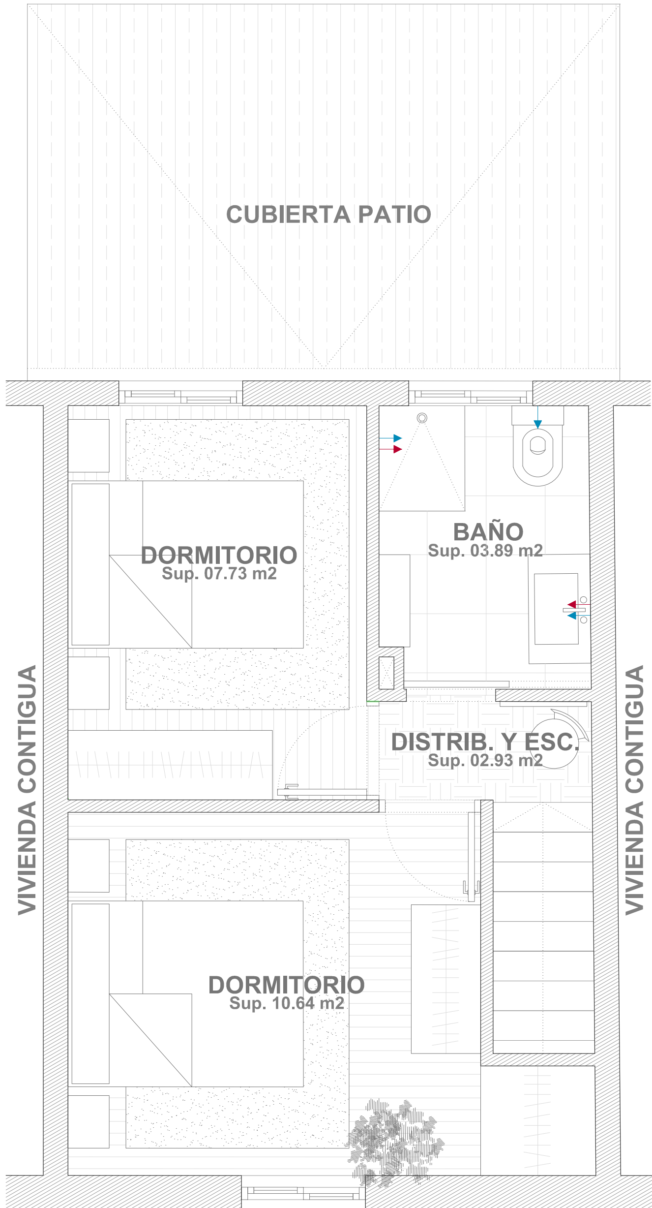
PLANTA PRIMERA
