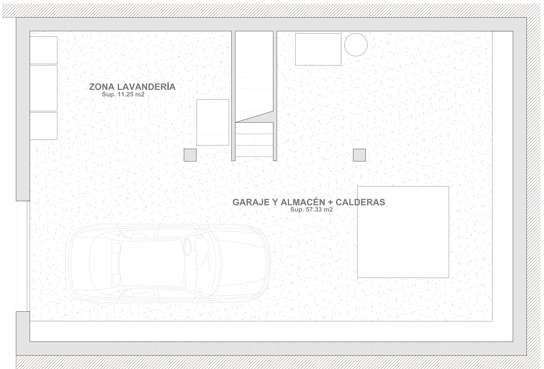
PLANTA SEMISÓTANO
